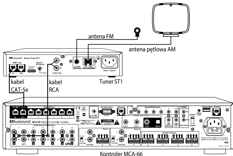
Połączenie MCA-66 ze źródłem RNET
