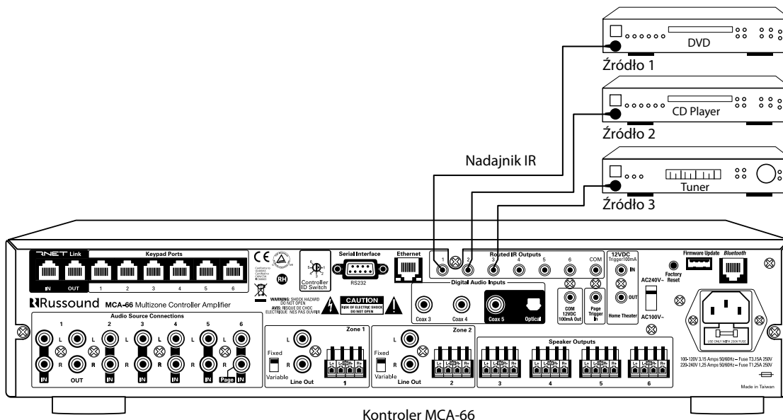
Połączenie podczerwieni (IR) z MCA-66
