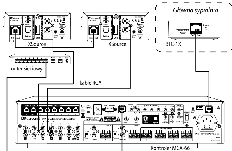
Połączenie MCA-66 ze źródłem audio
