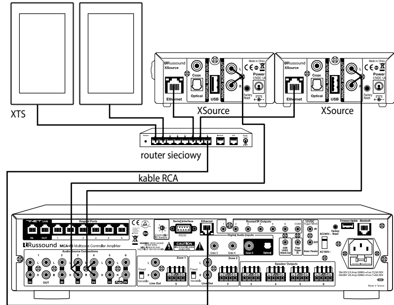
Połączenie XTS z MCA-66
