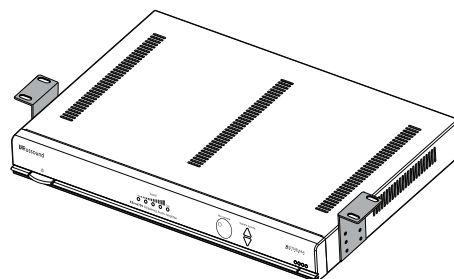
Montaż pod powierzchnią Przymocuj załączone uchwyty montażowe do obu stron sprzętu, z otworami montażowymi zwróconymi ku górze, jak pokazano na rysunku powyżej.
