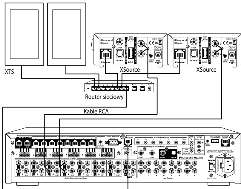
Połączenie XTS z MCA-88X
