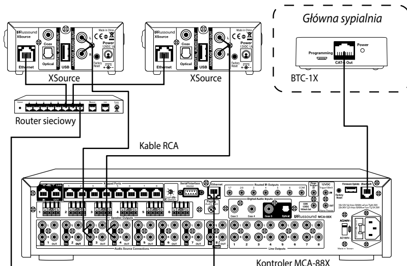
Połączenie MCA-88X ze źródłem audio
