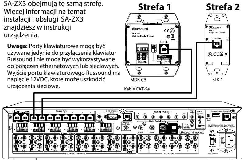
Połączenie klawiatury z MCA-88X
