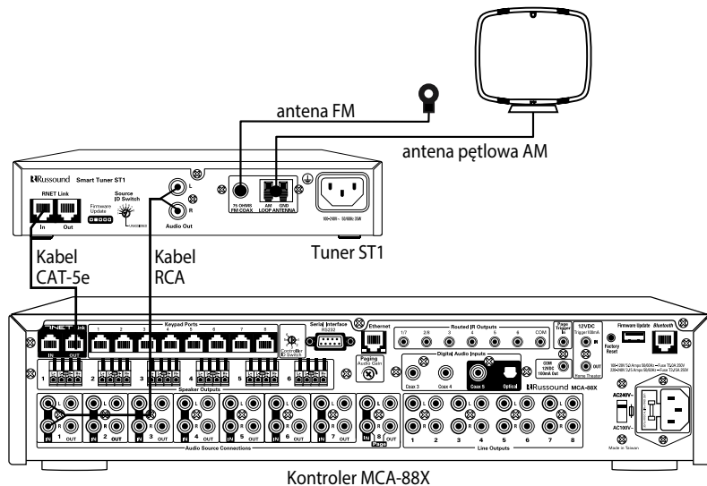
Połączenie MCA-88X ze źródłem RNET
