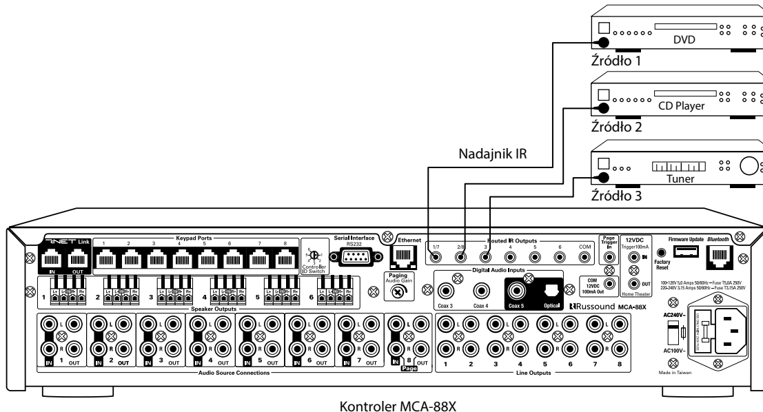
Połączenie podczerwieni (IR) z MCA-88X
