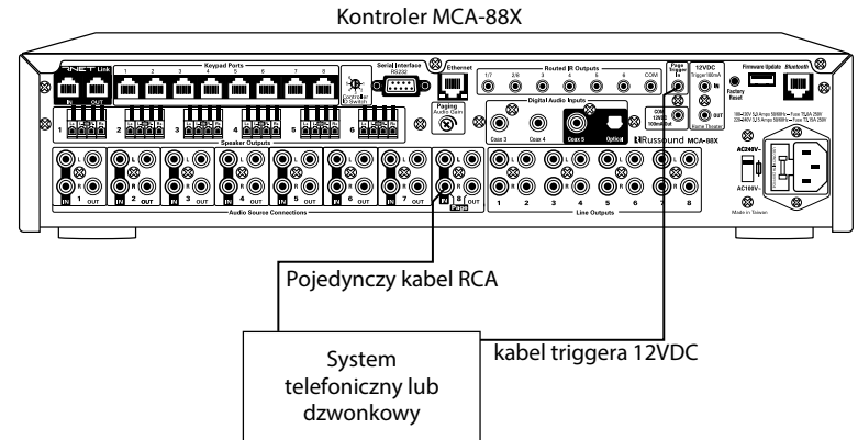
Typowa konfiguracja paging'u (przy użyciu Źródła nr 8 do zadań paging'owych)
