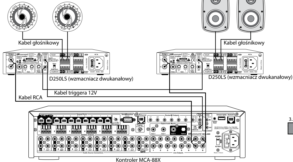
Typowe przyłączenie wzmacniacza
